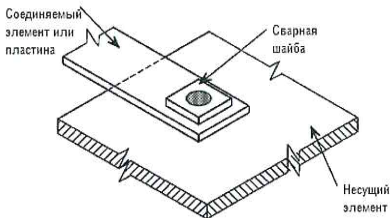
Рисунок 10.3 – Дуговая точечная сварка со сварной шайбой
