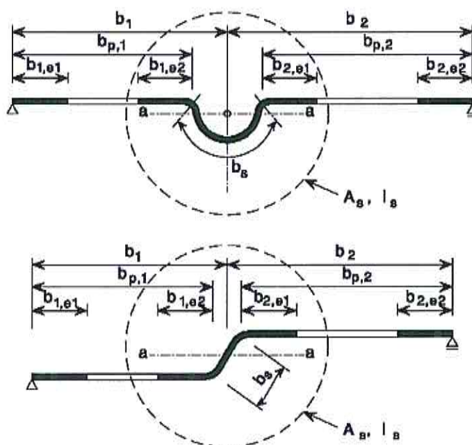
Рисунок 7.9 – Промежуточные элементы жесткости
