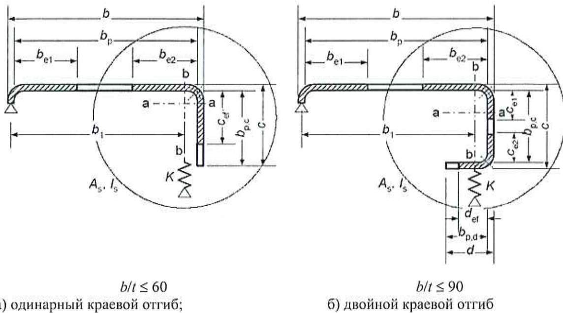
Рисунок 7.8 – Краевые отгибы
