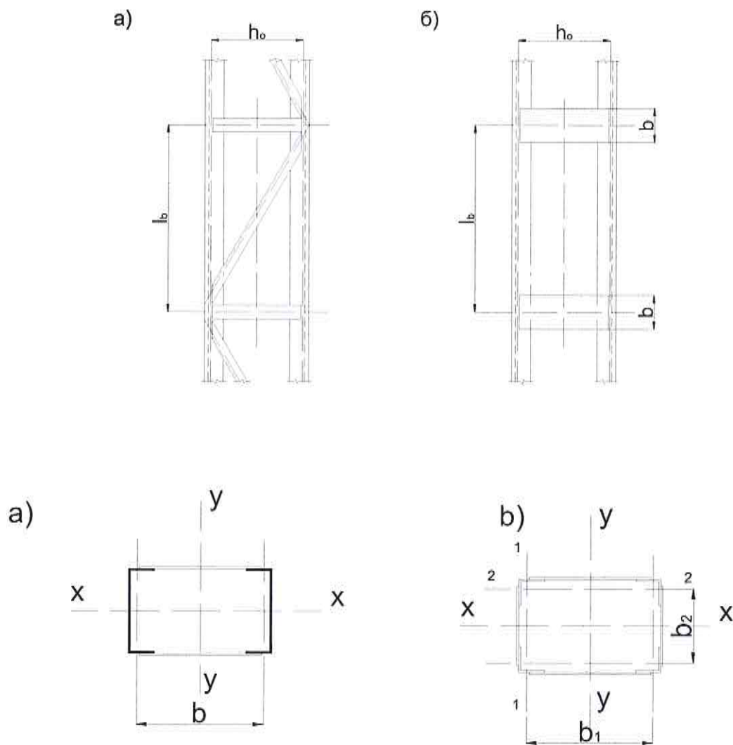
а) двухветвевая стержень
