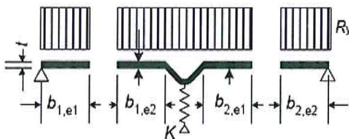
Рисунок Б.8 – Схема к этапу I. Эффективные ширины полки при \sigma_{com} = R_y
