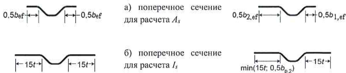
Рисунок 7.10 – Включение в ребро жесткости примыкающих участков полки
