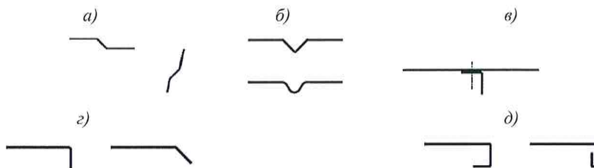
а) отгибы и сгибы; б) изогнутый или скругленный промежуточный элемент жесткости; в) уголок жесткости, присоединенный болтом; г) одиночные краевые отгибы; д) двойные краевые отгибы профилированных листов
